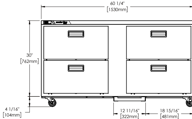
ELEVATION
